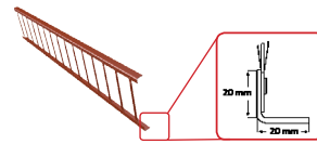
Gitterschenkelmaß
